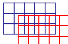
Subpixel-Verschiebung
