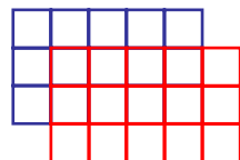
ganzzahlige Verschiebung
