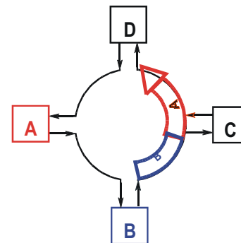
4. B ergreift Token und überträgt Rahmen B
