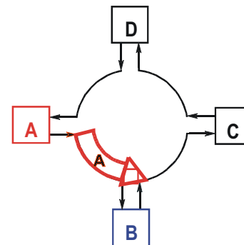
2. A ergreift Token und überträgt Rahmen A
