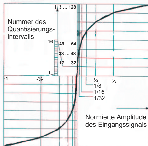
13-Segment-Kompressorkennlinie
