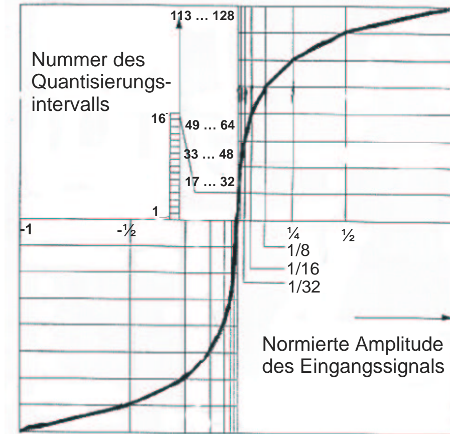
13-Segment-Kompressorkennlinie
